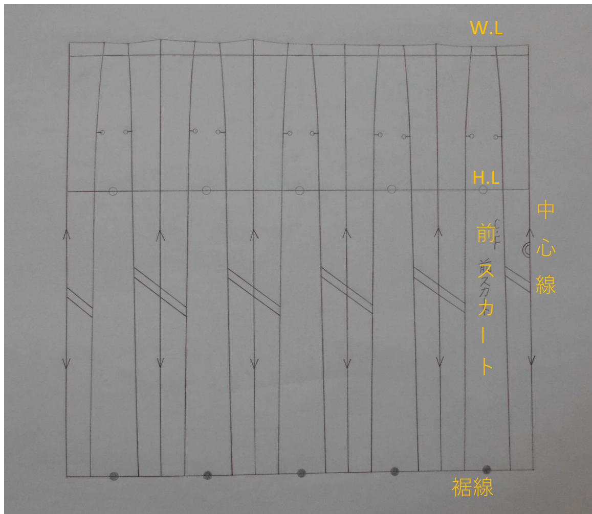
[プリーツのパターン展開]
